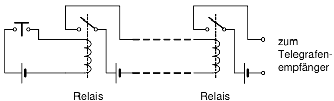
Bild 1.1.: Verstärkung digitaler Signale mit Hilfe elektromagnetischer Relais
