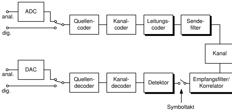
Bild 1.2.: Signalübertragung im Basisband
