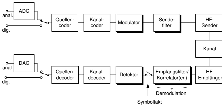
Bild 1.3.: Signalübertragung im Bandpassbereich (modulierte Signalübertragung)
